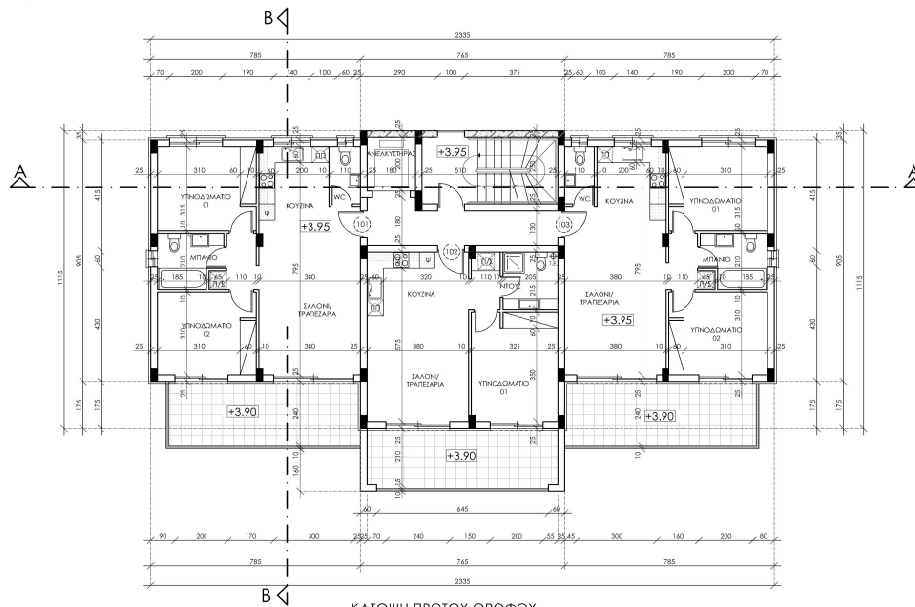
ΚΑΤΩΦΗ ΠΡΩΤΟΥ ΟΡΟΦΟΥ BLOCK D
