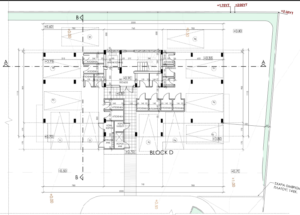
ΚΑΤΩΦΗ ΙΣΟΓΕΙΟΥ / ΠΛΑΤΗΣ BLOCK D
