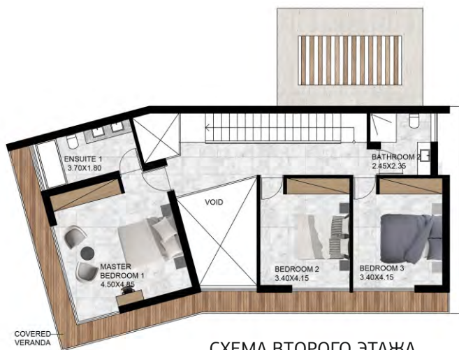
СХЕМА ВТОРОГО ЭТАЖА
