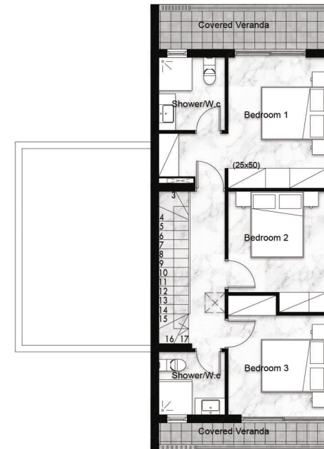
СХЕМА ВТОРОГО ЭТАЖА
