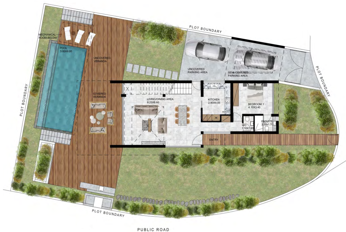
СХЕМА ПЕРВОГО ЭТАЖА
