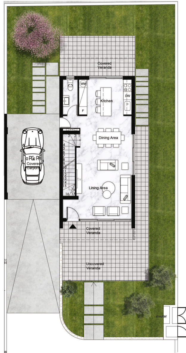
СХЕМА ПЕРВОГО ЭТАЖА
