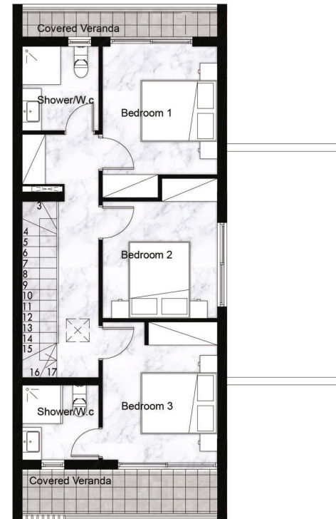
СХЕМА ВТОРОГО ЭТАЖА
