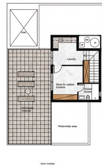
ПЛАН КРЫШИ С САДОМ
