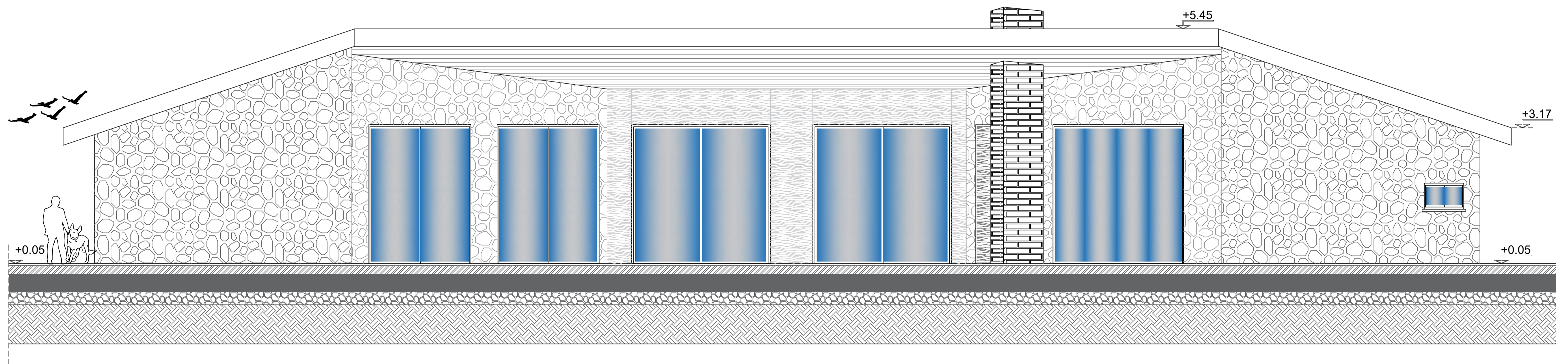
ΠΡΟΣΩΠΗ- ΚΥΡΙΑ ΚΑΤΟΙΚΙΑ ΚΛΙΜΑΚΑ 1/50
