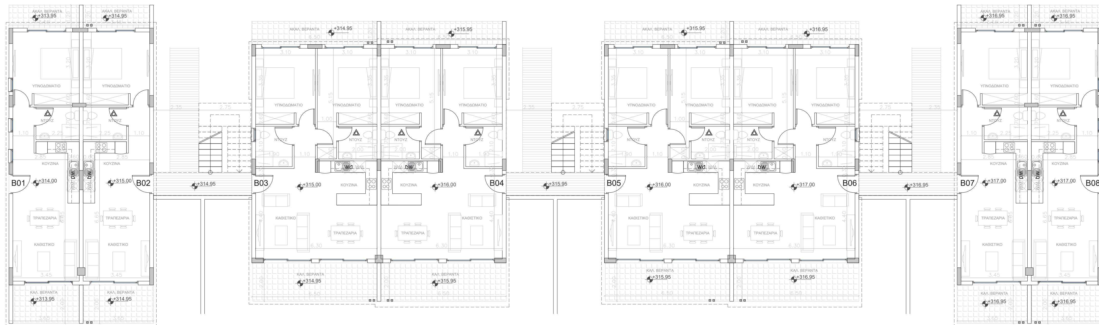
BLOCK B - ΚΑΤΟΨΗ ΙΣΟΓΕΙΟΥ
